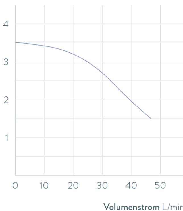
PUMPENKENNLINIEN Temperierflüssigkeit: Wasser Standardpumpe, 60 Hz Druck bar
