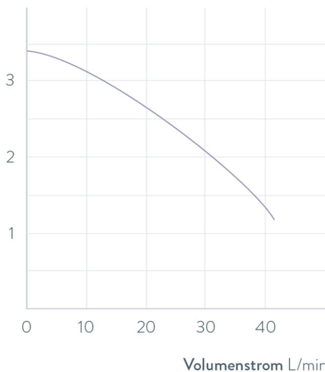
PUMPENKENNLINIEN Temperierflüssigkeit: Wasser Standardpumpe, 50 Hz Druck bar
