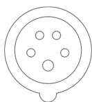
Câble secteur avec fiche (IEC 60309, 5-pol, CEE, rouge, 16 A)
