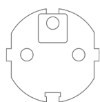
Cable de alimentación con conector Schuko (CEE7/7)
