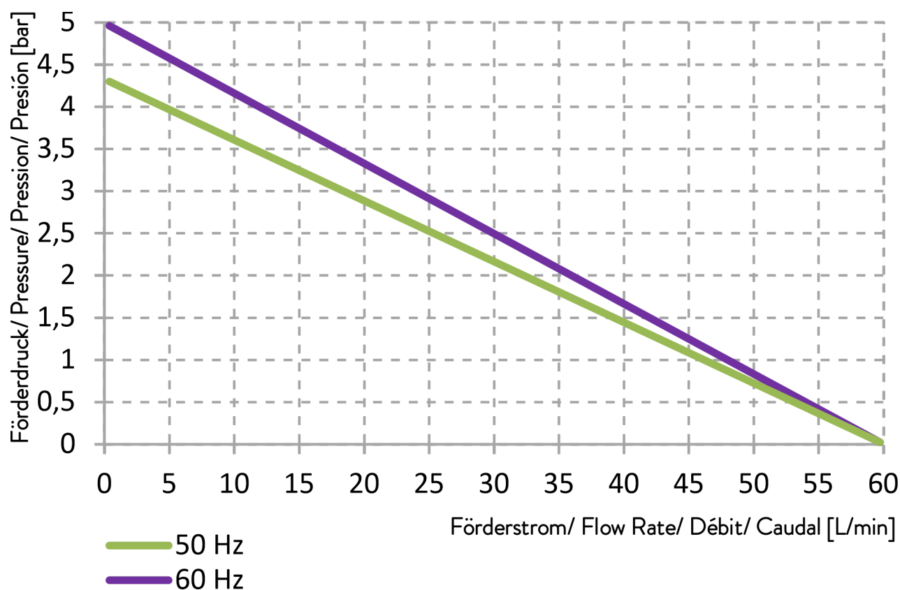
Fig. 77: Curvas características de la bomba
