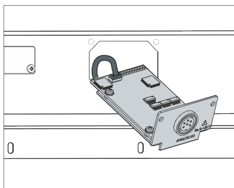
Fig. 19: Conector en el casquillo
