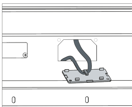
Fig. 18: Cable enganchado en la tapa
