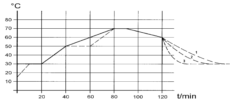
Fig. 62: Programa de ejemplo
