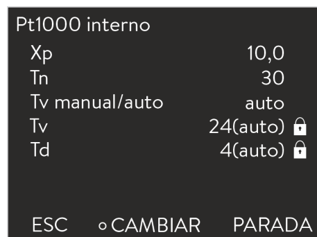
Fig. 44: Menú Parámetros de regulación internos
