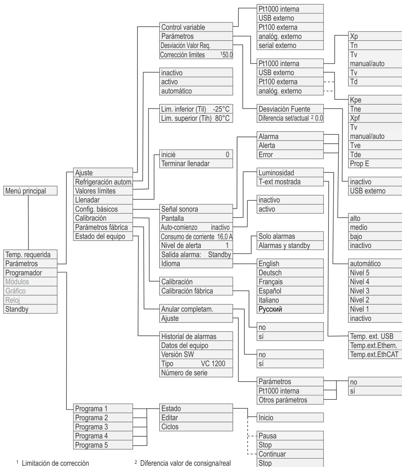
Fig. 20: Estructura del menú, parte 1
