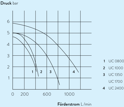
PUMPENKENNNLINIEN Flüssigkeit: Wasser
