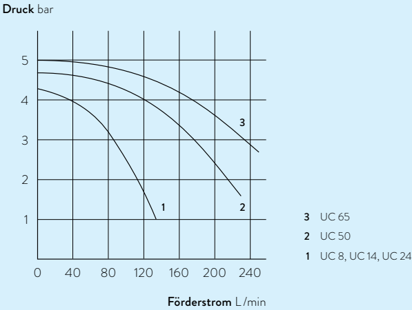
PUMPENKENNNLINIEN Flüssigkeit: Wasser
