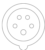
Netzkabel mit Stecker (IEC 60309, 5-pol, CEE, rot, 32 A)
